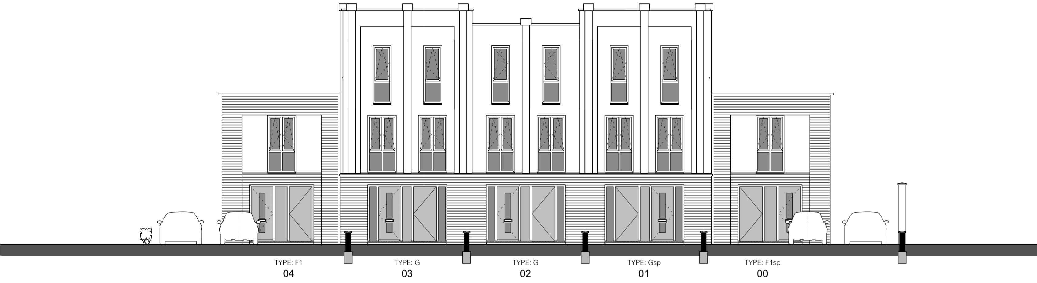
Vooraanzicht schaal 1:100
